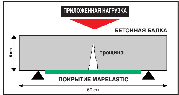
Рис. 1: Защита с помощью Mapelastic волосяной трещины с нижней стороны балки, подверженной давлению на изгиб
